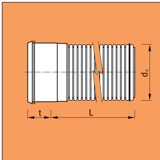
Прага канализационная труба из ПП, двойные стенки
